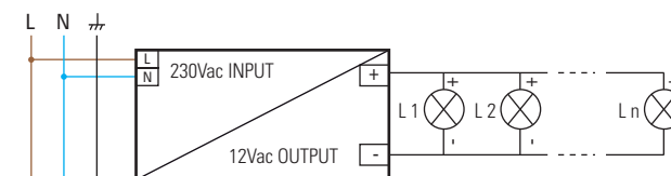
Schéma de câblage
