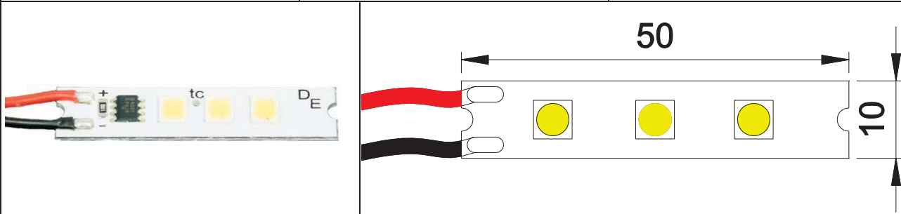
LED-Leiterplatte für Konstantspannung LED PCB for constant voltage
